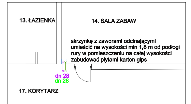
SZCZEGÓŁ "B"
